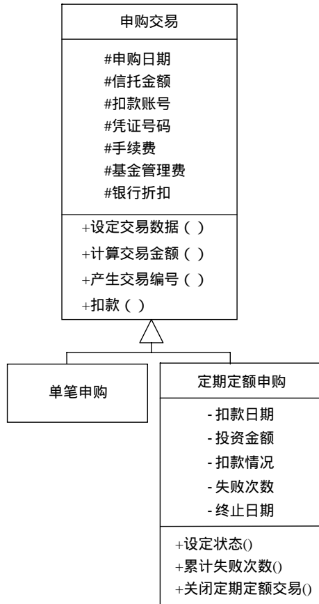
图10-22 泛化关系
