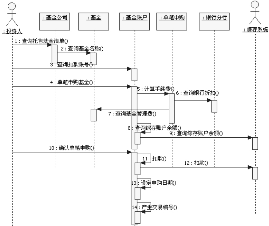
图10-31 建立11~14号消息
