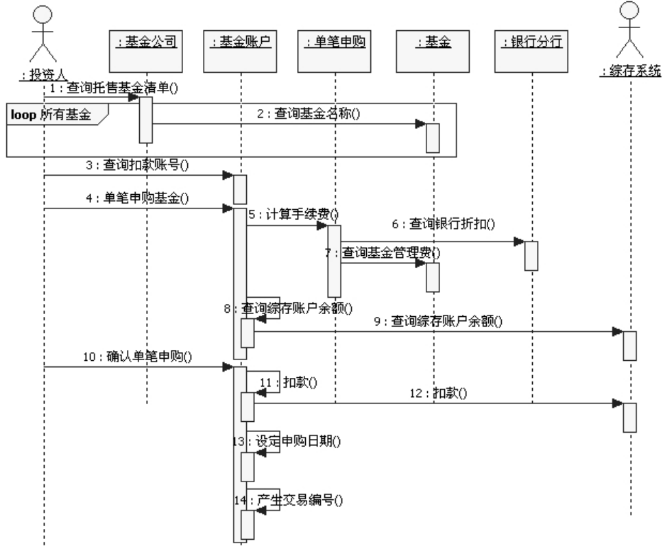
图10-32 调整序列图
