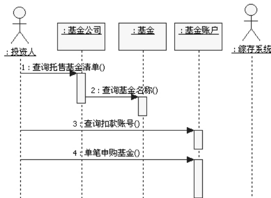
图10-27 建立4号消息
