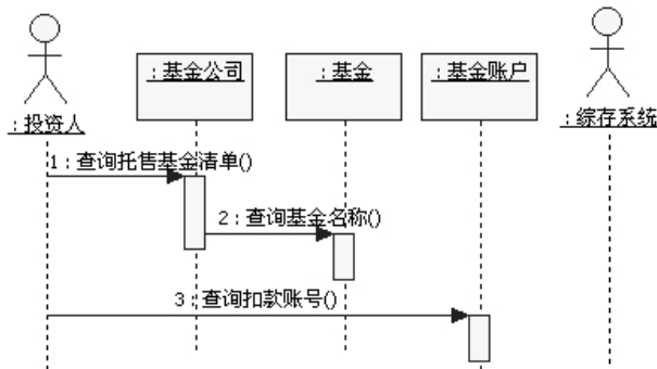
图10-26 建立1~3号消息
