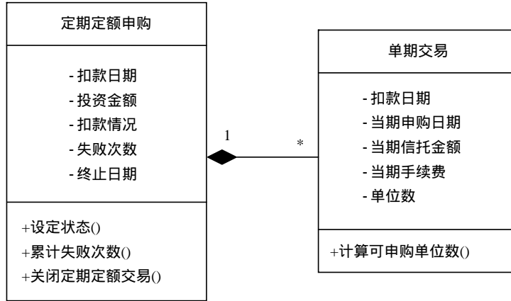
图10-23 组合关系
