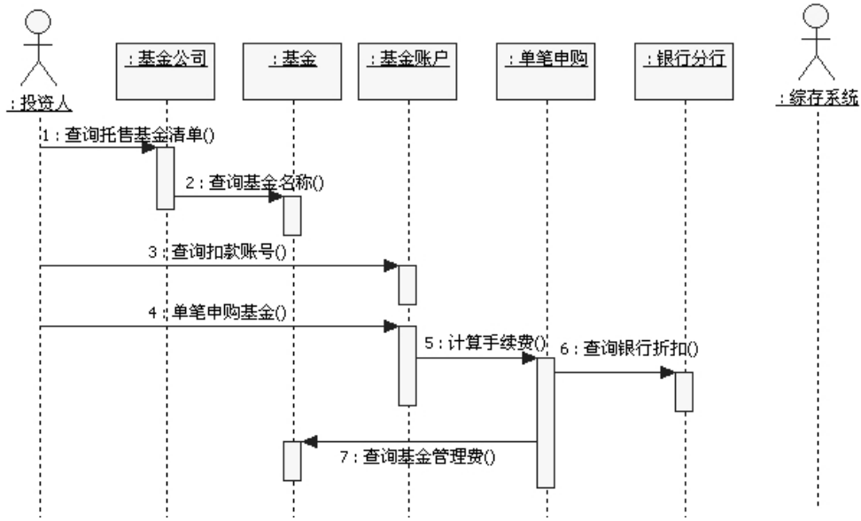
图10-28 建立5~7号消息
